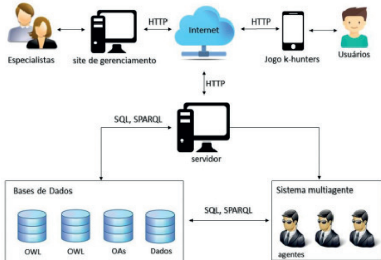
Figura 2: Arquitetura do K-hunters
