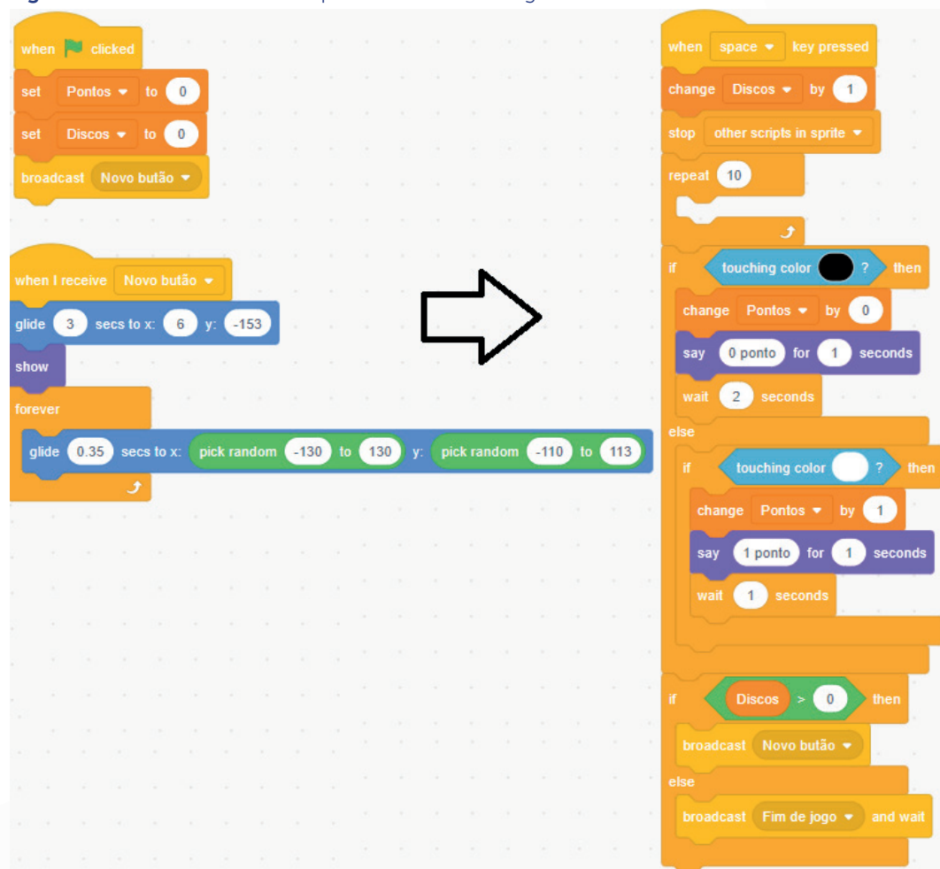
Figura 2 – Entrada de comandos por meio de blocos lógicos do Scratch.
