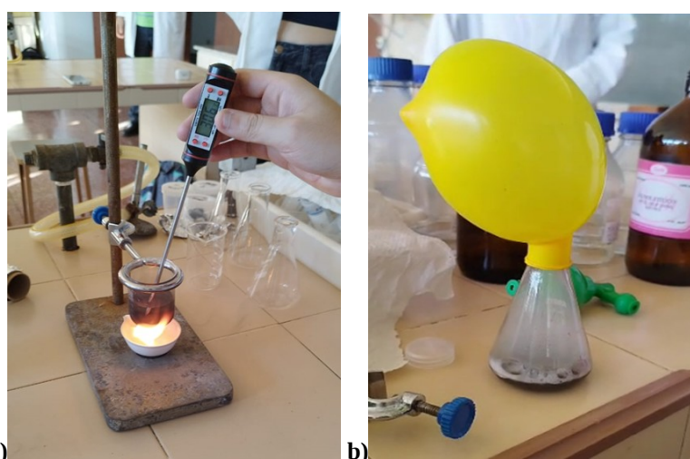
Figura 2: Montagem e testagem do experimento de combustão proposto na oficina Fonte: Autores (2025)
