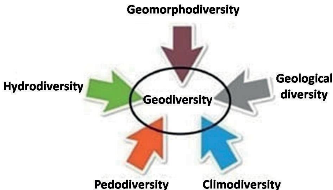
Figura 1. A Geodiversidade e seus elementos integrantes (Fonte: Claudino-Sales, 2021)
