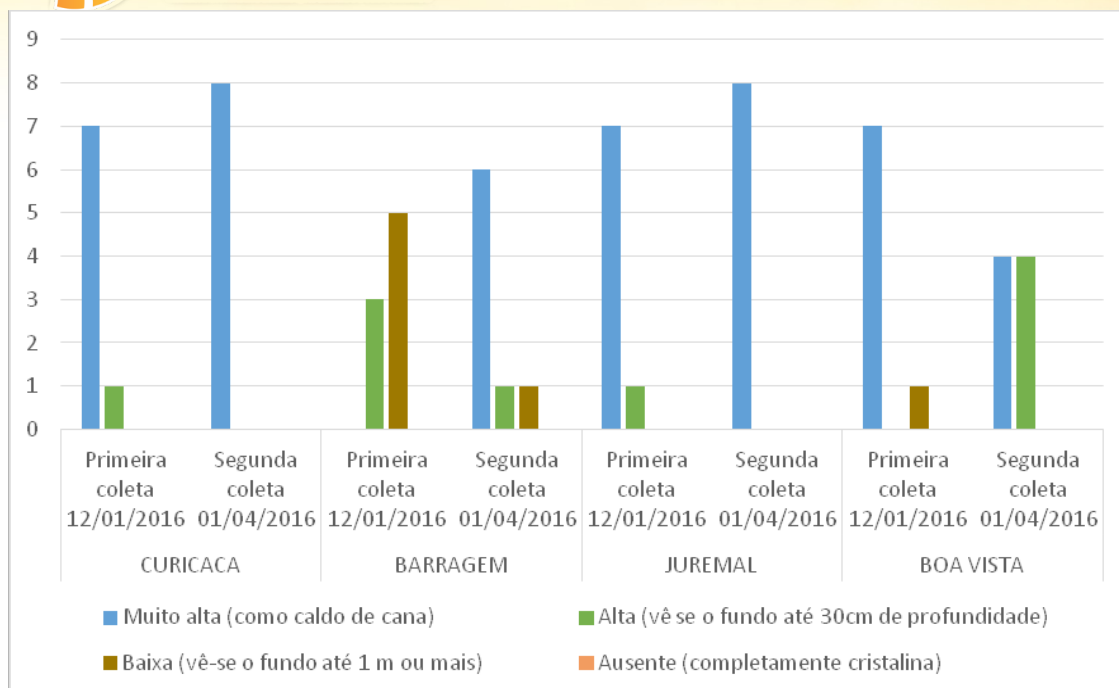
Figura 02: Avaliação da turbidez em quatro pontos ao longo do rio Potengi e no entorno da barragem Campo Grande/RN.
