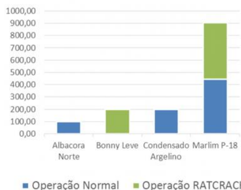
Figura 5: Volume destilado em cada campanha.
