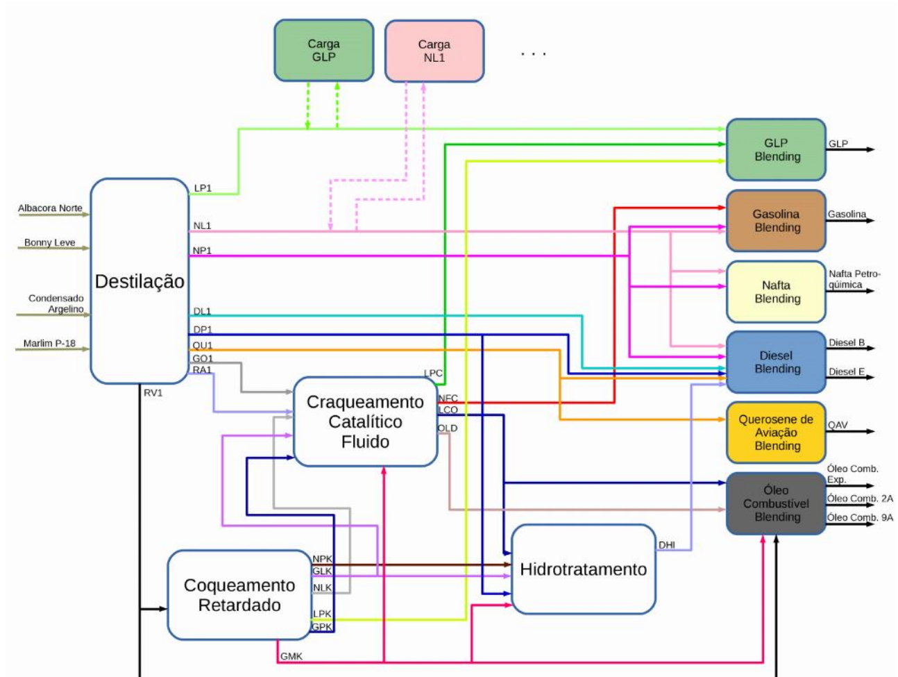
Figura 2: Modelo da refinaria.
